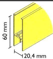
Horizontalus profilis, L-6000, Aliuminio arba šampano spalvos
