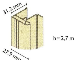
Rankenėlės profilis, L-2700, Aliuminio arba šampano spalvos
